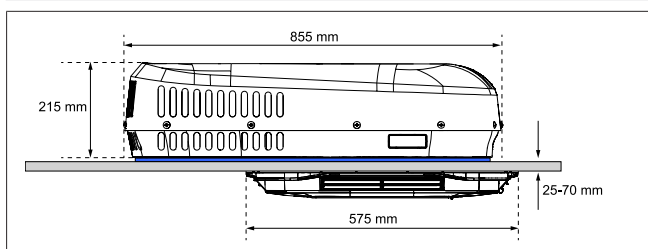
Abb. 7 Einbaumaße (Seitenansicht)
