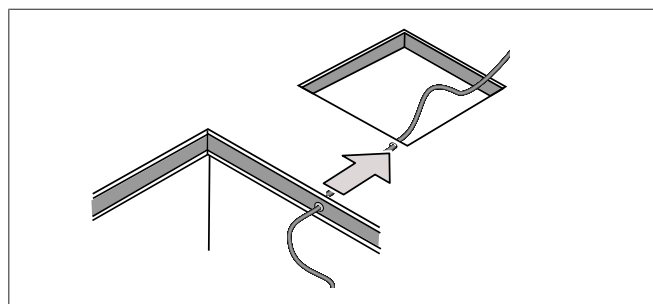
Fig. 12 Cavo CI-BUS
