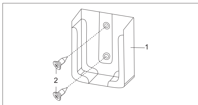
Fig. 32 Supporto telecomando
