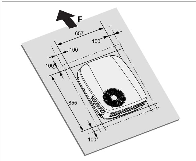
Fig. 5 Direzione di installazione dell'unità esterna
