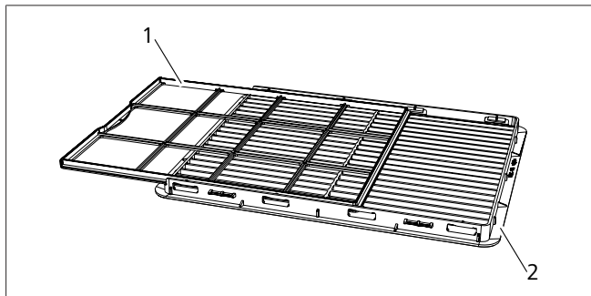
Fig. 56 Filtro dell'aria
