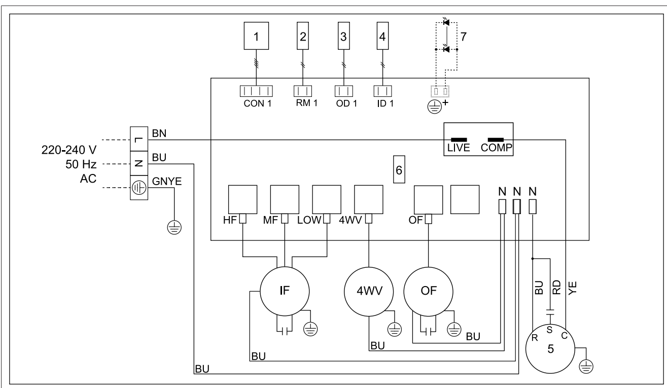
Afb. 58 Bedradingsschema
