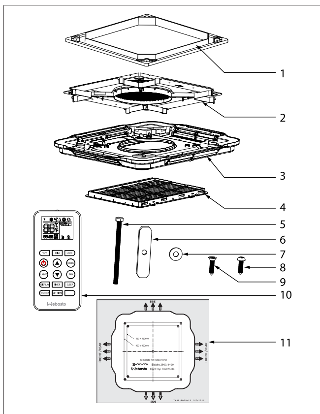
Fig. 2 Unità interna
