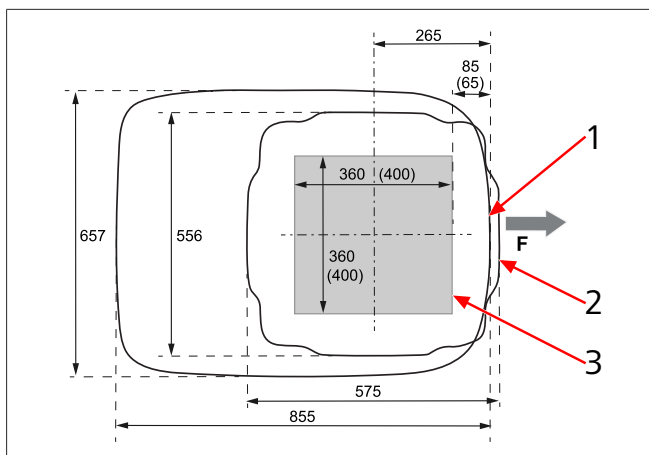
Bild 6 Monteringsmått (vy uppifrån/nerifrån)
