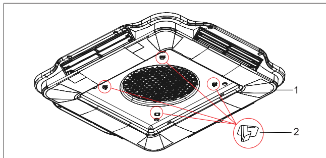
Fig. 28 Conexión del conjunto de distribuidor de aire al soporte de montaje
