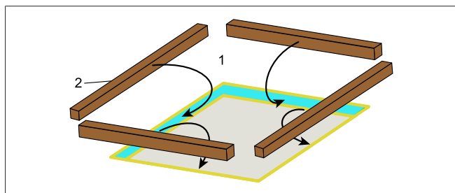
Fig. 9 Rinforzo tetto
