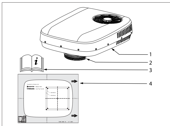
Fig. 1 Unità esterna
