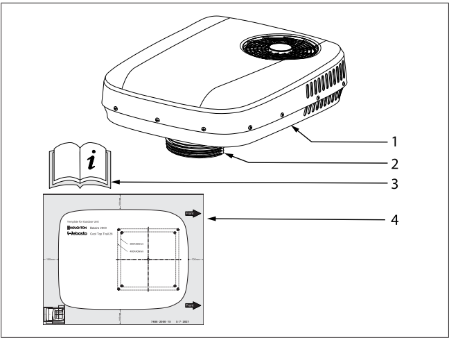
Fig. 1 Unité extérieure
