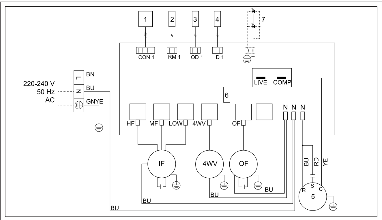
Fig. 58 Schema elettrico
