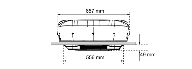
Bild 8 Monteringsmått (vy framifrån)
