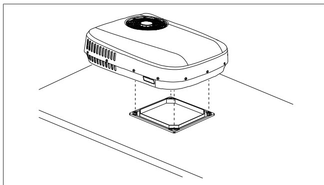
Abb. 18 Positionieren der Außeneinheit
