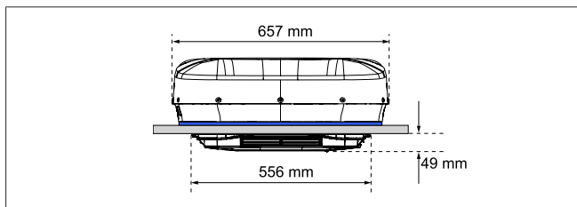
Afb. 8 Montage-afmetingen (vooraanzicht)
