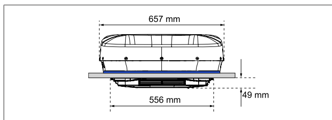
Fig. 8 Misure installazione (vista frontale)
