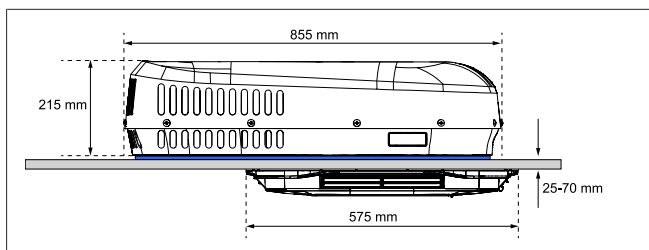
Afb. 7 Montage-afmetingen (zij-aanzicht)
