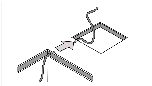
Afb. 11 Kabel elektrische externe voeding
