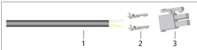
Bild 13 Montering CI-BUS-kabel
