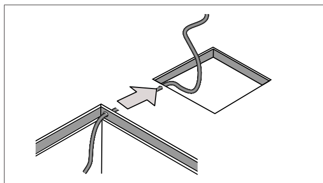
Bild 11 Strömförsörjningskabel
