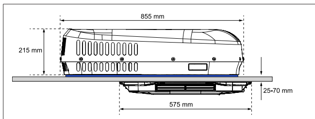
Fig. 7 Medidas de montaje (vista lateral)
