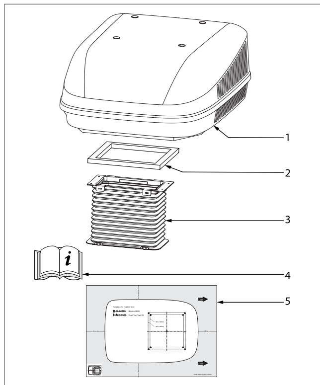
Abb. 1 Außeneinheit
