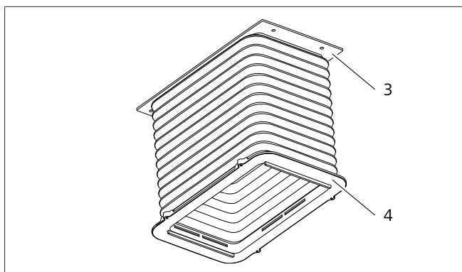
Abb. 19 Zuluftkanal
