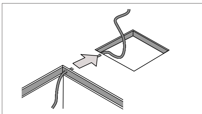
Afb. 9 Kabel elektrische externe voeding
