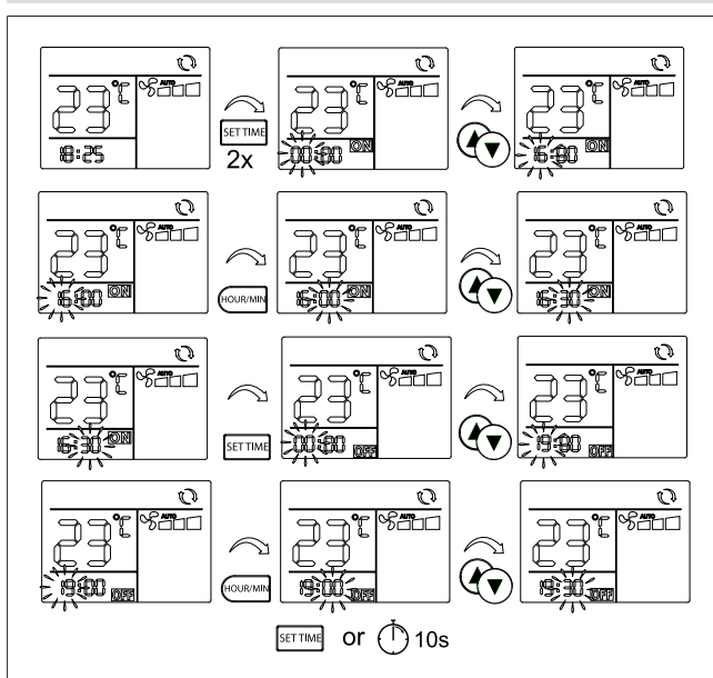
Fig. 41 Réglage de la minuterie
