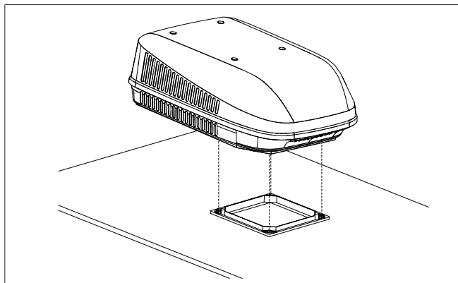
Afb. 16 De buiteneenheid plaatsen
