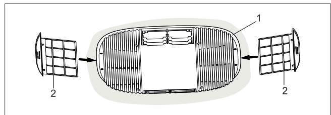
Abb. 27 Einbau der Luftfilter
