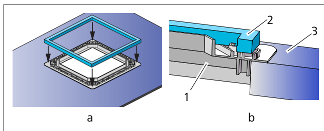
Fig. 13 Montaje de la junta en un bastidor adaptador (recorte de tamaño 400 x 400)
