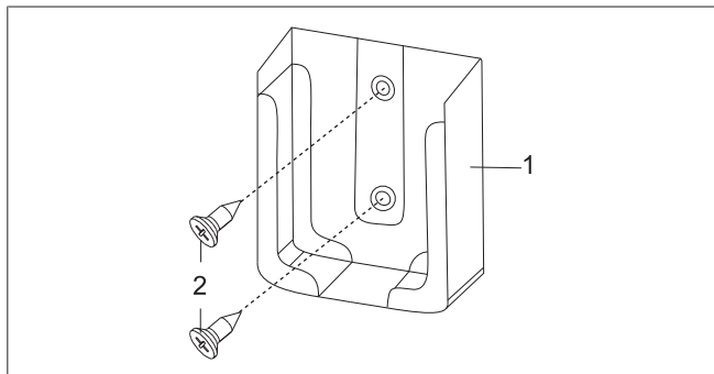
Bild 28 Fjärrkontrollens hållare
