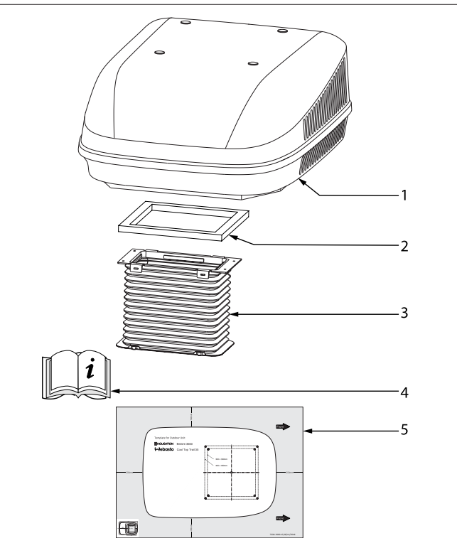
Fig. 1 Unité extérieure
