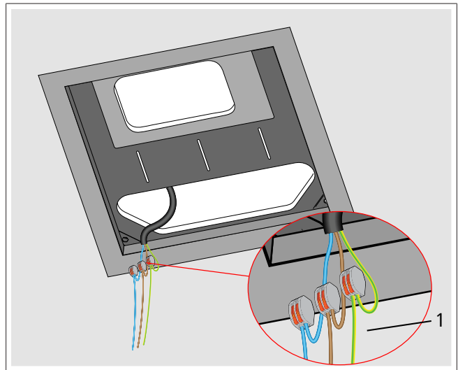
Abb. 17 Position der Klemmleisten
