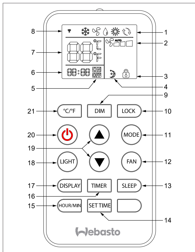
Fig. 29 Panoramica telecomando
