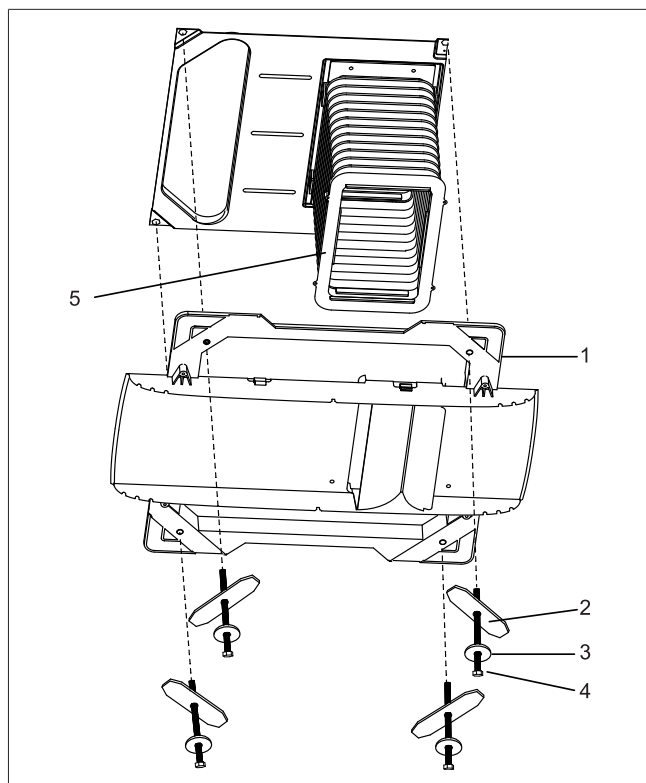
Afb. 20 De bouten monteren
