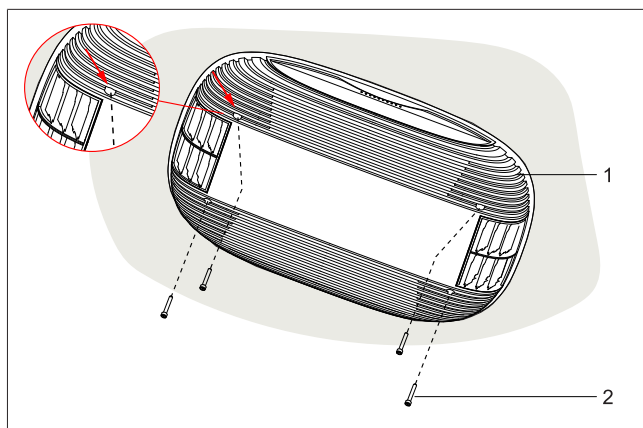
Bild 25 Fästa luftfördelarenheten på monteringskonsolen
