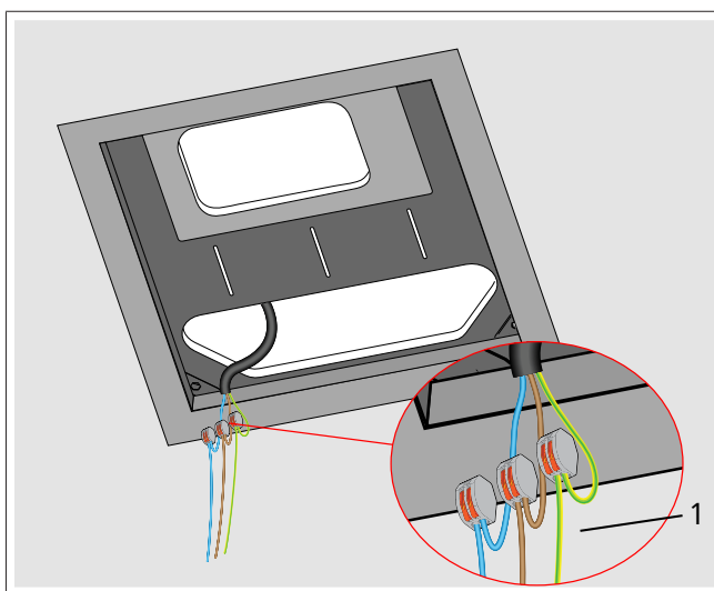
Bild 17 Kopplingsplintarnas placering
