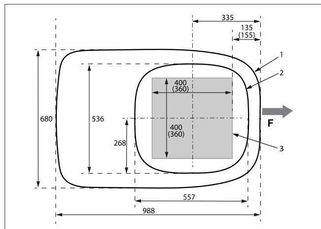
Fig. 4 Mesures pour l'installation (vue du haut/de dessous)
