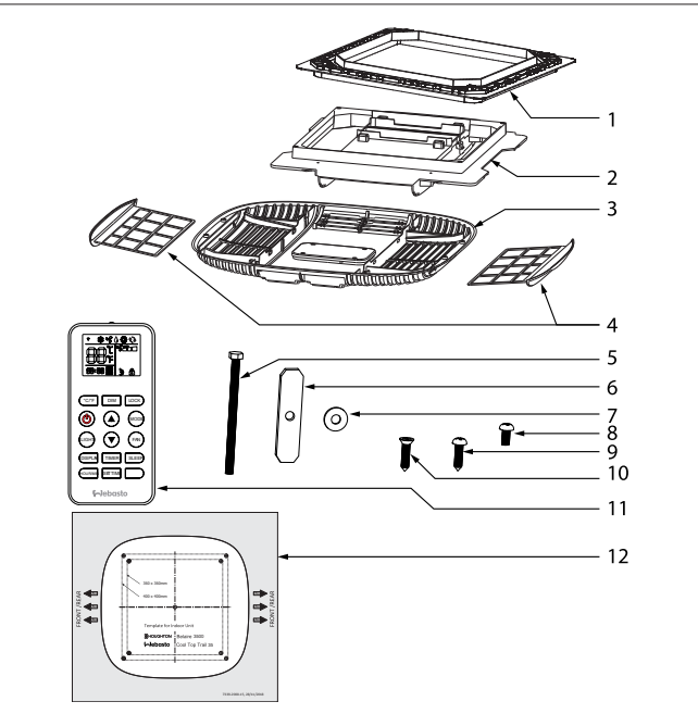
Fig. 2 Unidad interior
