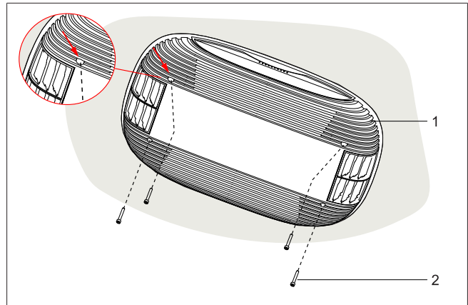
Abb. 25 Befestigen des Luftverteilers an der Halterung
