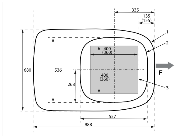
Abb. 4 Einbaumaße (Ansicht von oben/unten)
