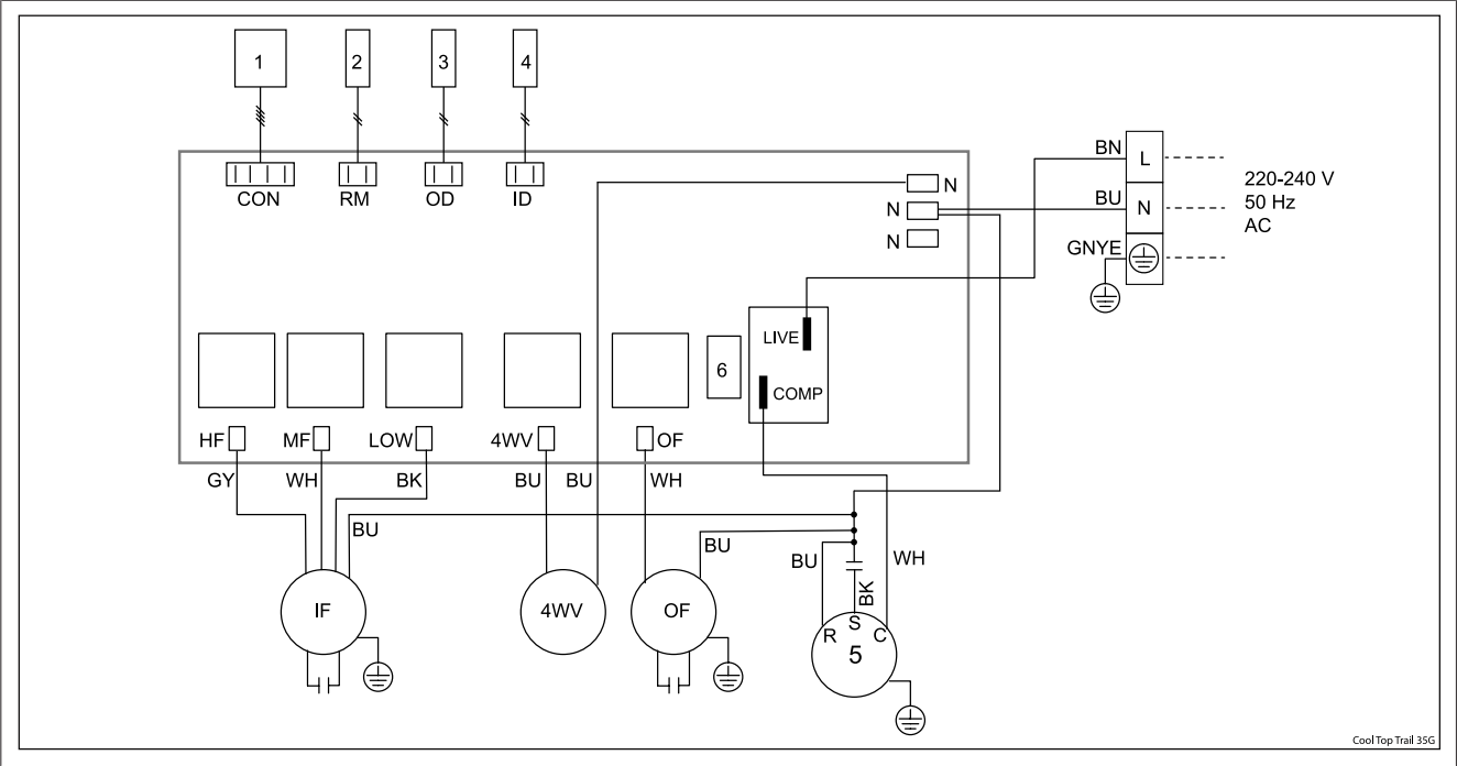
Fig. 53 Esquema eléctrico
