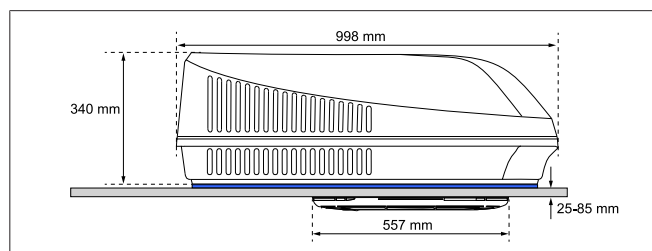
Afb. 5 Montage-afmetingen (zij-aanzicht)
