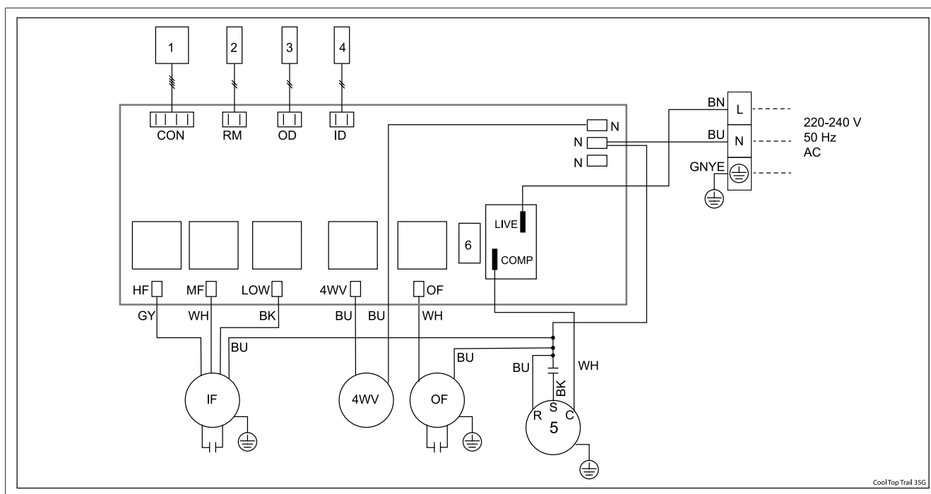
Afb. 53 Bedradingsschema
