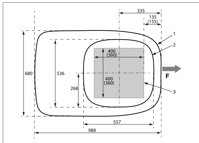
Afb. 4 Montage-afmetingen (boven-/onderaanzicht)
