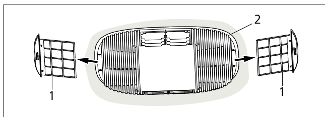
Fig. 51 Démontage des filtres à air
