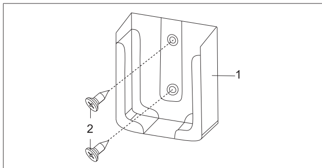
Afb. 28 Houder afstandsbediening
