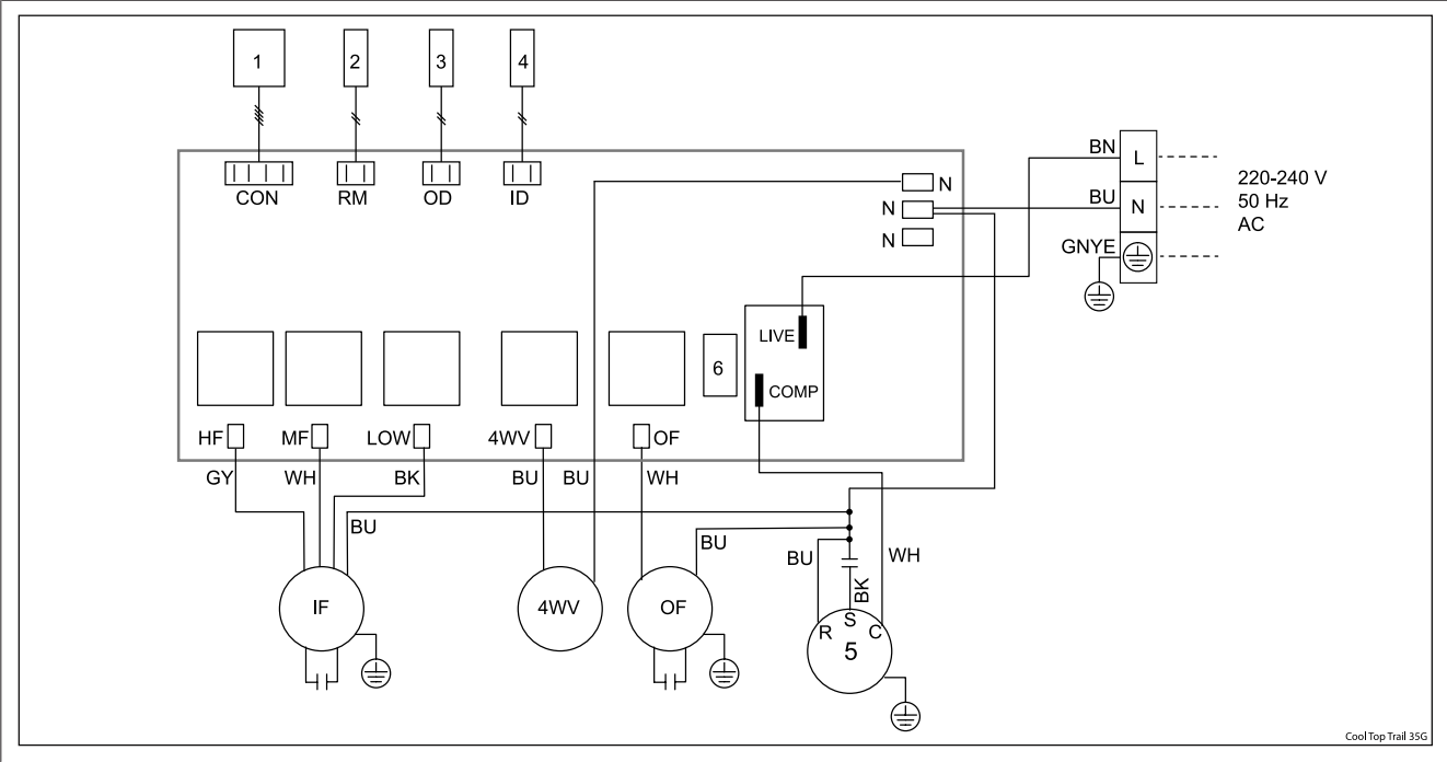
Fig. 53 Schéma électrique
