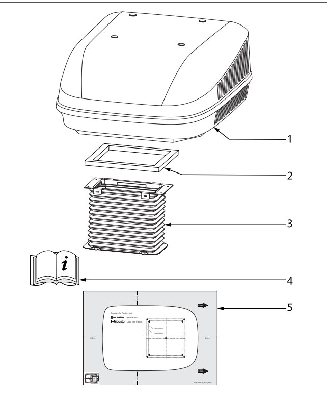
Fig. 1 Unidad exterior
