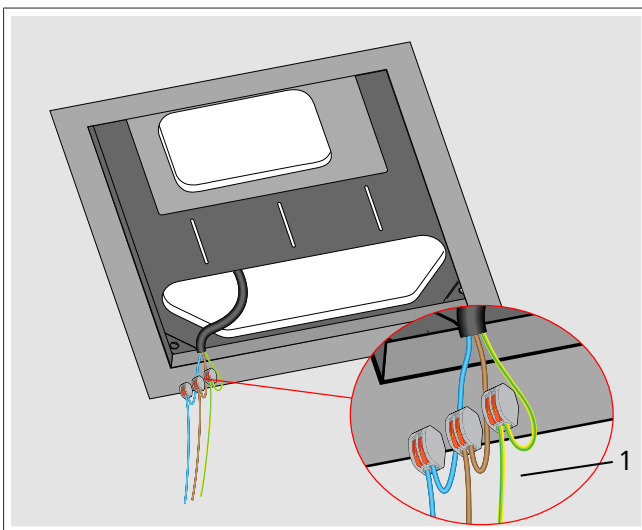
Afb. 17 Locatie van de aansluitblokken
