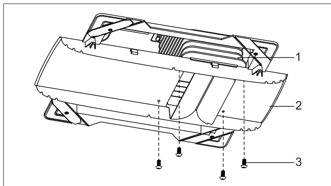
Fig. 21 Conexión del conducto de salida de aire
