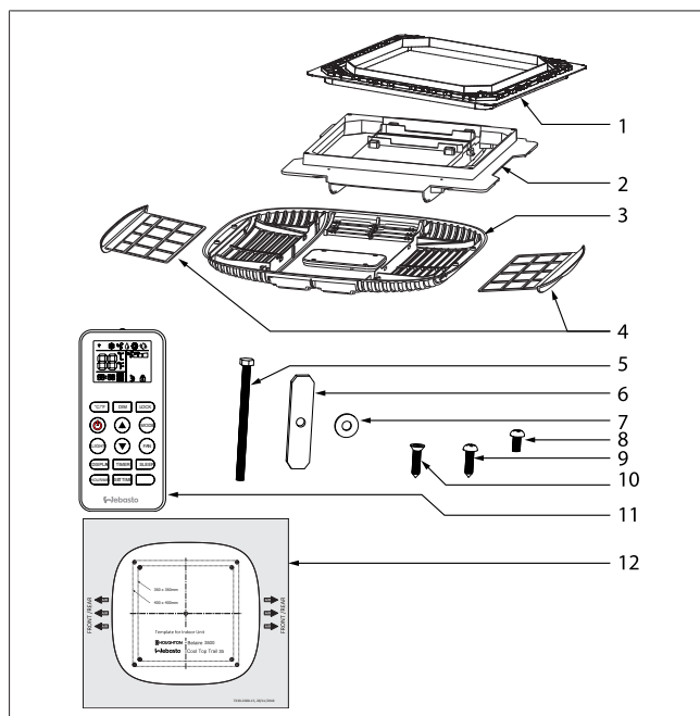
Abb. 2 Inneneinheit
