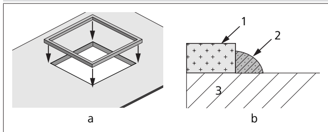
Bild 14 CTT35_Montering_av_packningen på en 360 x 360-utskärning (utan adapterram)
