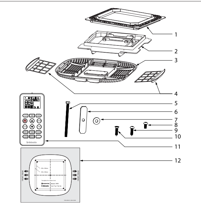
Fig. 2 Unité intérieure
