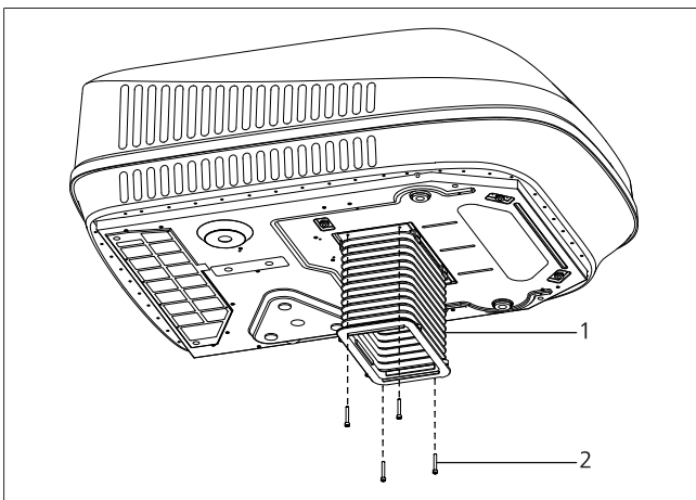
Afb. 18 Het luchtinlaatkanaal installeren
