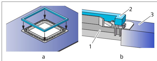
Fig. 13 Montage du joint sur un cadre adaptateur (découpe 400 x 400)
