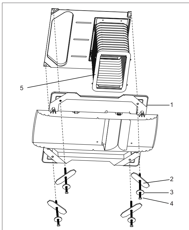
Fig. 20 Instalación de los pernos
