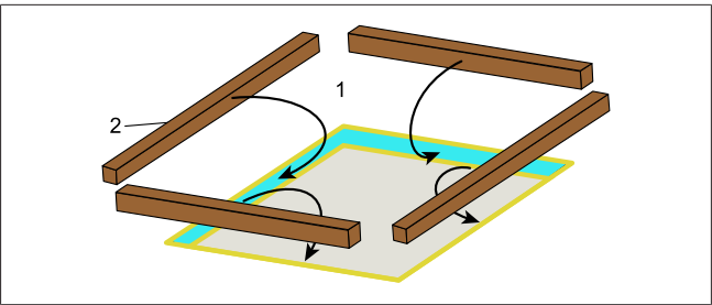
Fig. 7 Rinforzo tetto
