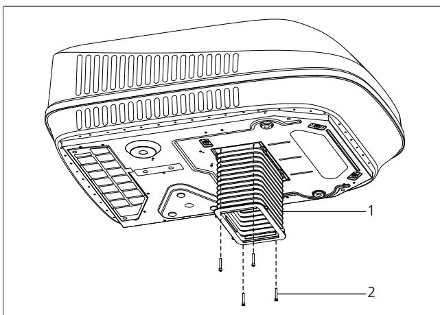
Fig. 18 Installazione del condotto di ingresso dell'aria
