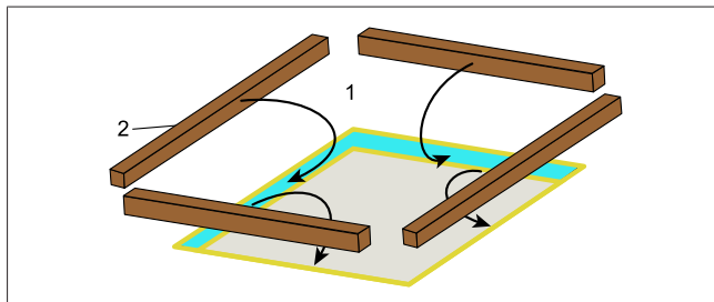
Abb. 7 Dachverstärkung
