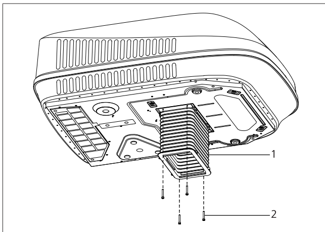
Bild 18 Montering av luftintagskanalen
