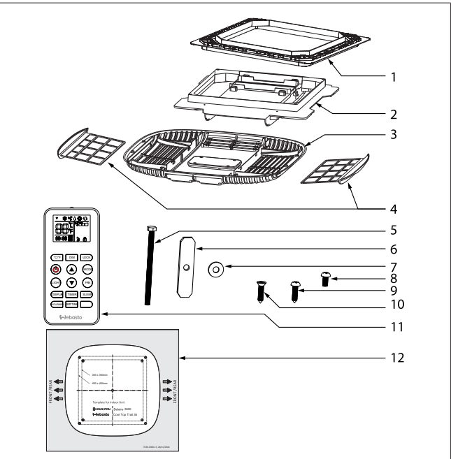
Fig. 2 Unità interna
