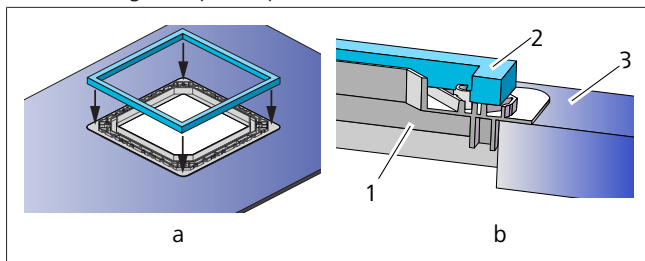
Bild 13 Montering av packningen på en adapterram (400 x 400 utskärning)
