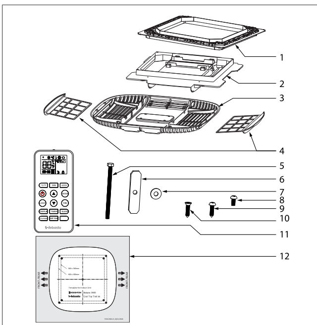
Afb. 2 Binneneenheid
