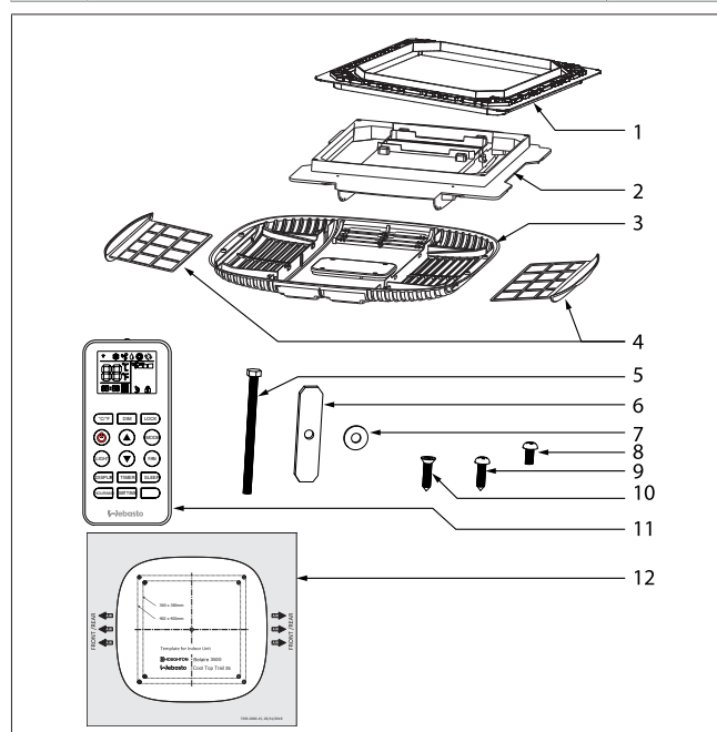
Bild 2 Inomhusenhet
