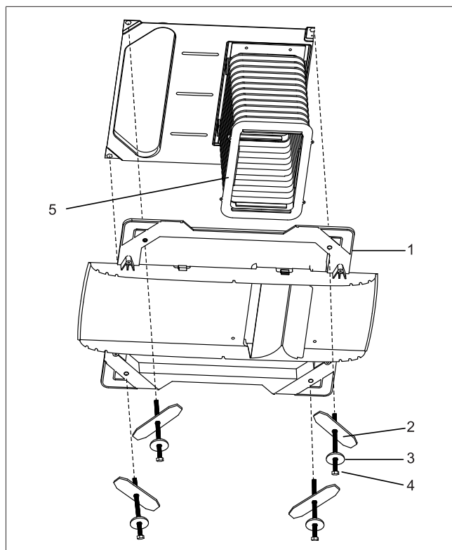
Abb. 20 Einsetzen der Schrauben
