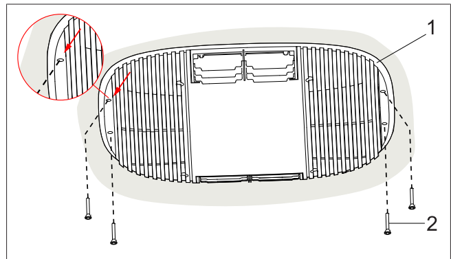
Abb. 26 Befestigen des Luftverteilers am Fahrzeugdach
