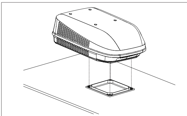
Abb. 16 Positionieren der Außeneinheit
