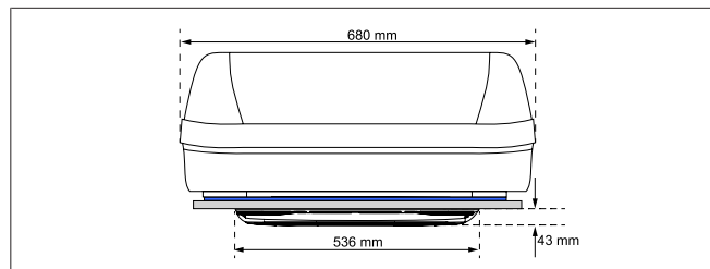
Afb. 6 Montage-afmetingen (vooraanzicht)
