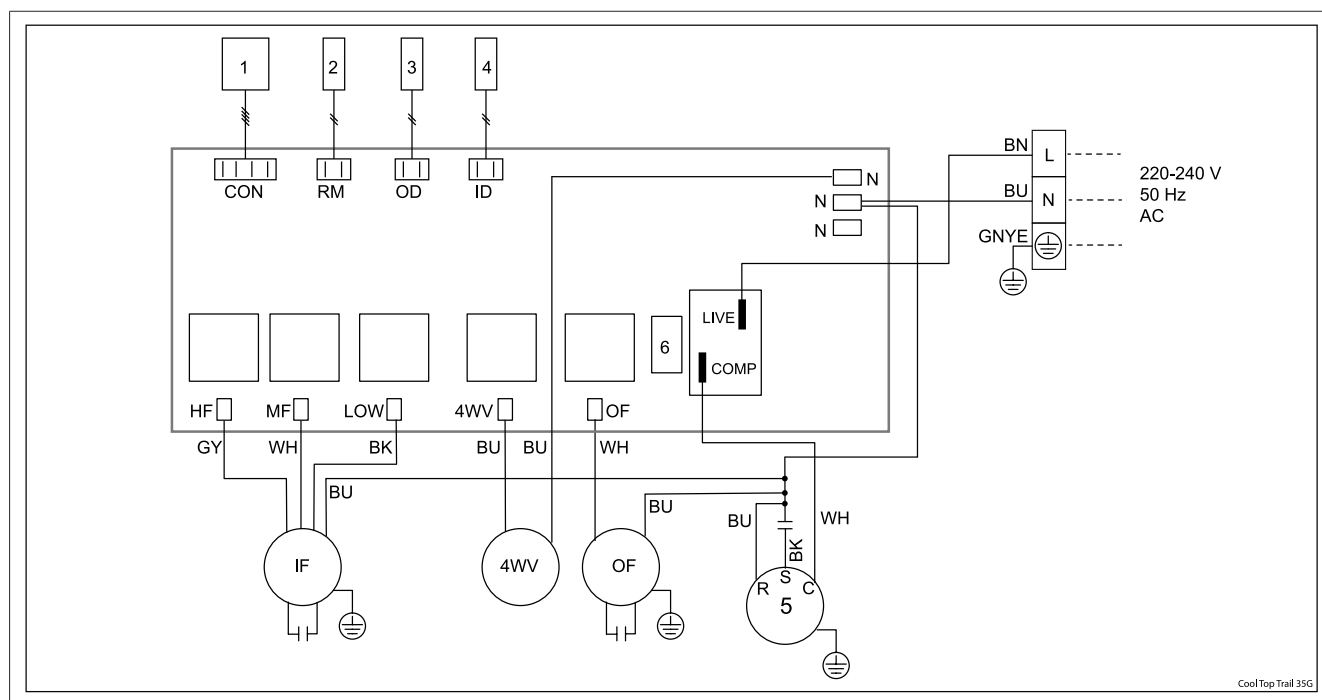
Bild 53 Systemkopplingsschema
