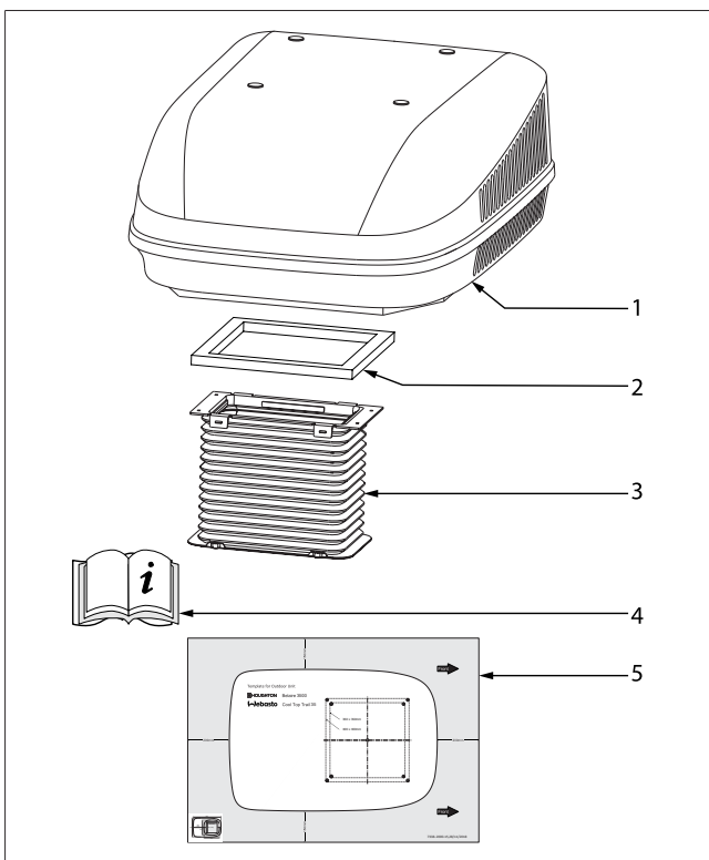
Afb. 1 Buiteneenheid
