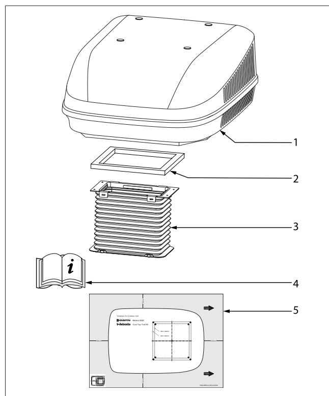
Bild 1 Utomhusenhet
