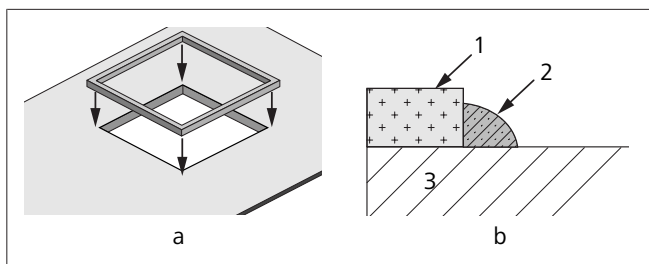
Afb. 14 CTT35_De_pakking_bevestigen op een 360 x 360 uitsnede (zonder adapterframe)
