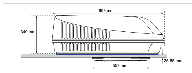
Abb. 5 Einbaumaße (Seitenansicht)
