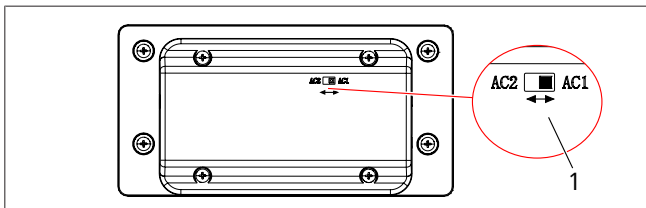
Afb. 25 Bovenaanzicht van de CI-BUS-eenheid
