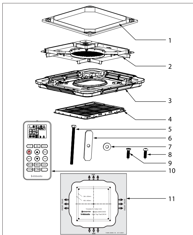
Fig. 2 Unité intérieure
