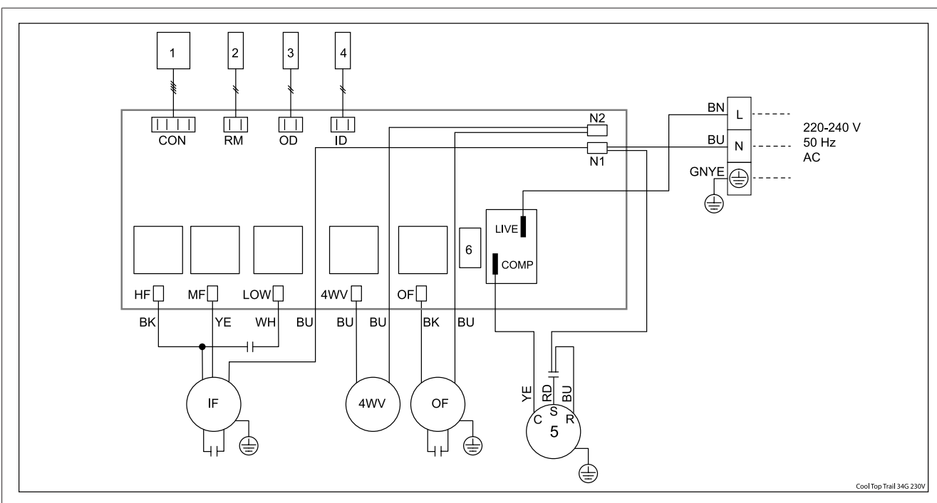
Afb. 58 Bedradingsschema
