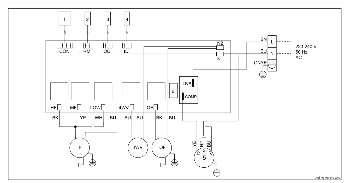
Fig. 58 Wiring diagram
