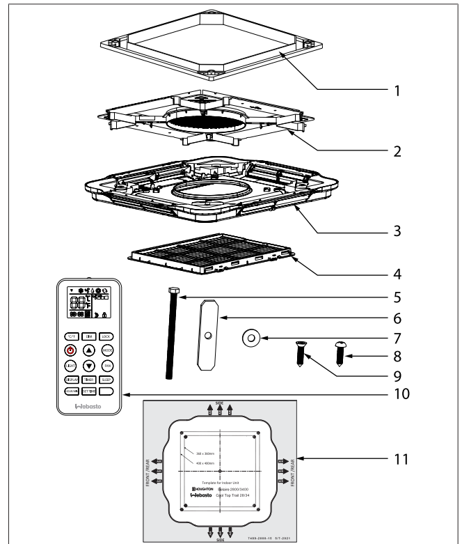
Fig. 2 Indoor unit
