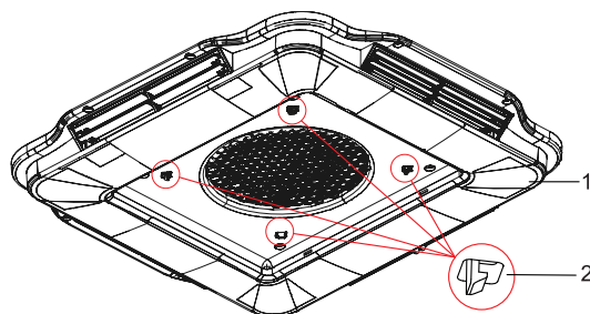
Fig. 28 Fixation du distributeur d'air sur le support de montage
