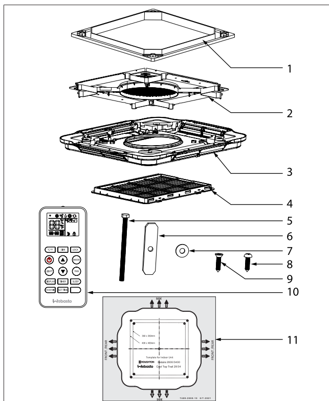
Abb. 2 Inneneinheit
