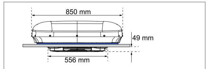
Bild 8 Monteringsmått (vy framifrån)
