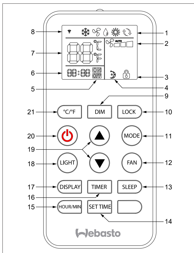
Fig. 33 Vista general del mando a distancia
