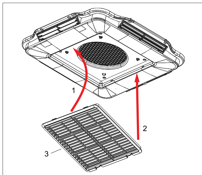
Fig. 31 Installation du filtre à air
