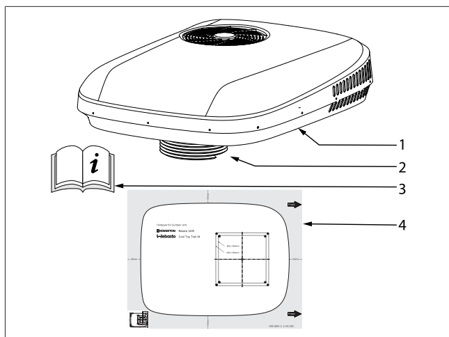
Bild 1 Utomhusenhet
