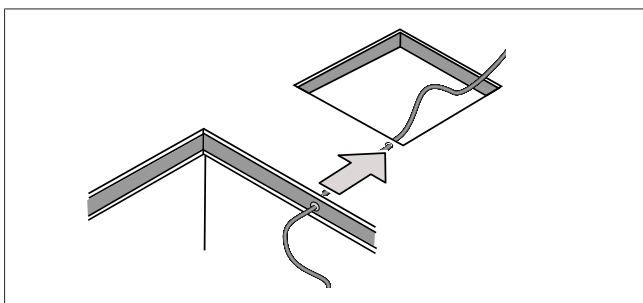
Fig. 12 Câble CI-BUS
