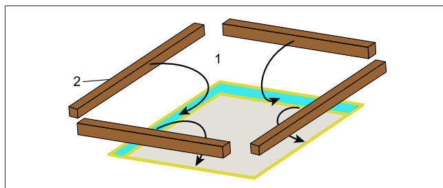
Fig. 9 Rinforzo tetto
