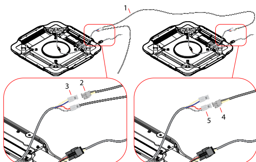
Fig. 26 Connexion de deux Unités CI-BUS
