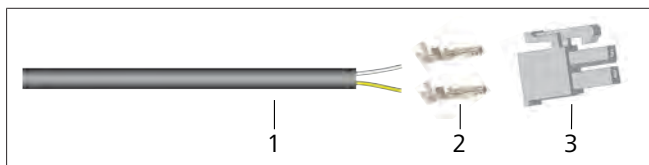
Abb. 13 Konfektionieren des CI-BUS-Kabels
