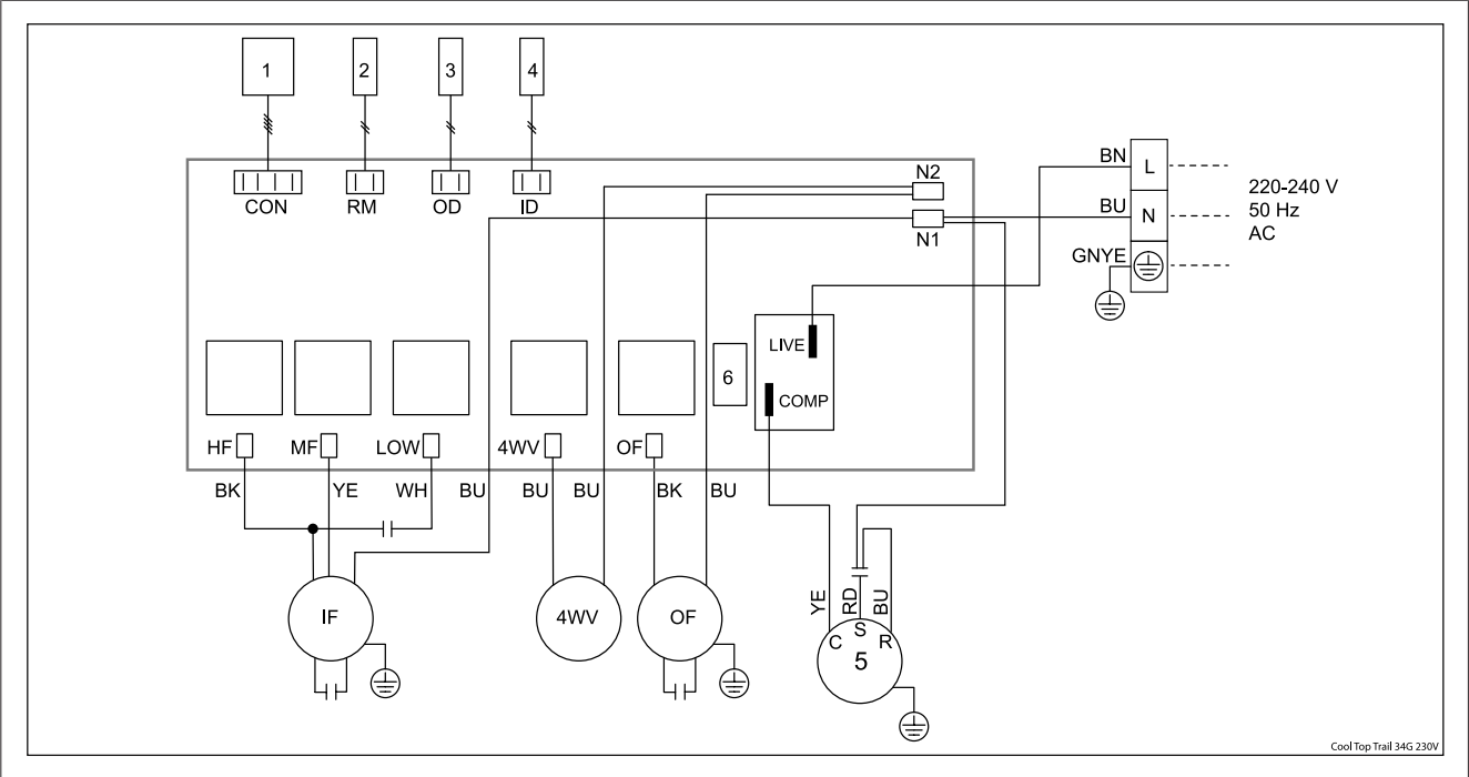
Fig. 58 Diagramma cablaggio
