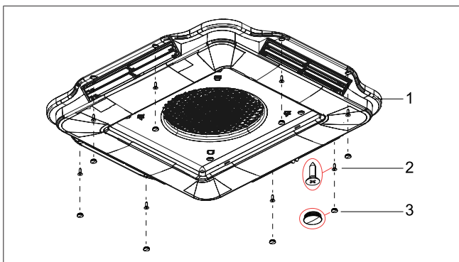
Abb. 30 Befestigen des Luftverteilers am Fahrzeugdach
