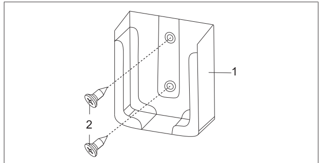
Afb. 32 Houder afstandsbediening
