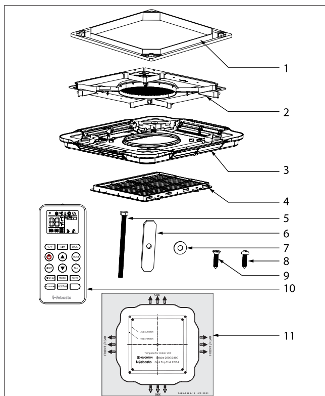
Fig. 2 Unità interna
