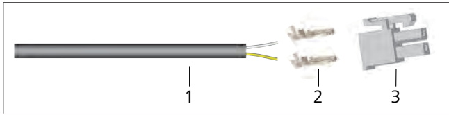
Afb. 13 Assemblage CI-BUS-kabel
