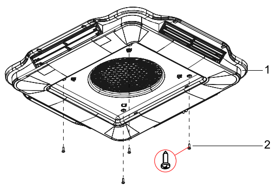
Fig. 29 Fixation du distributeur d'air sur le support de montage
