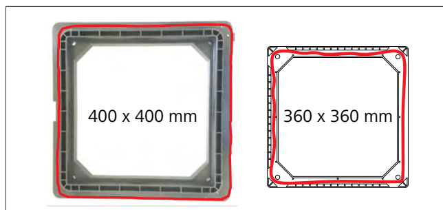
Abb. 16 Dichtungsverläufe
