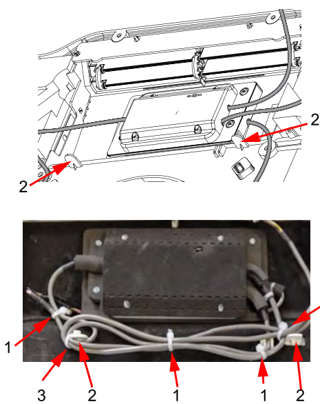
Fig. 27 Attacher les câbles
