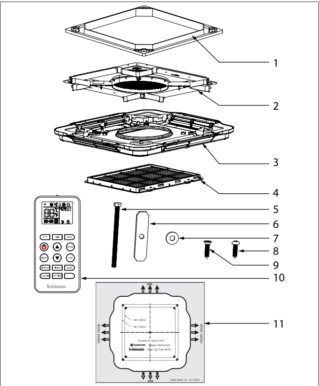
Fig. 2 Unidad interior
