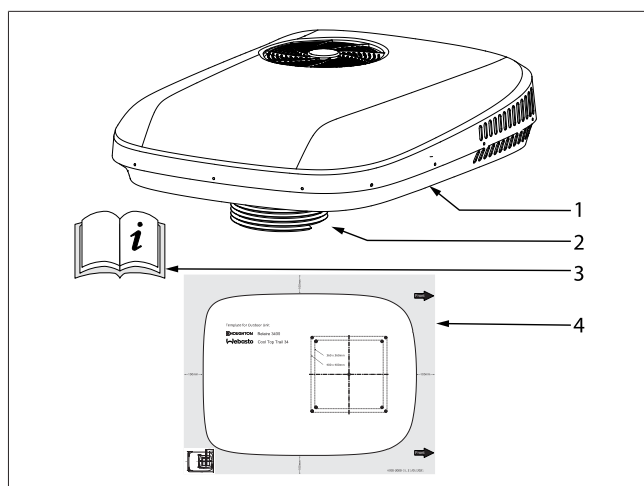
Fig. 1 Unità esterna
