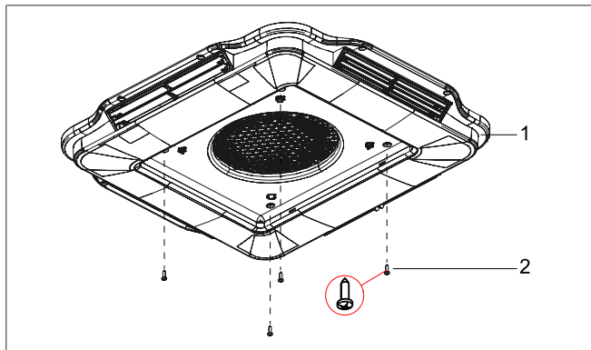
Fig. 29 Fissare il gruppo diffusore dell'aria alla staffa di montaggio
