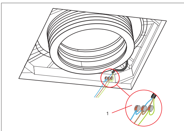
Fig. 19 Ubicación de los bloques de terminales
