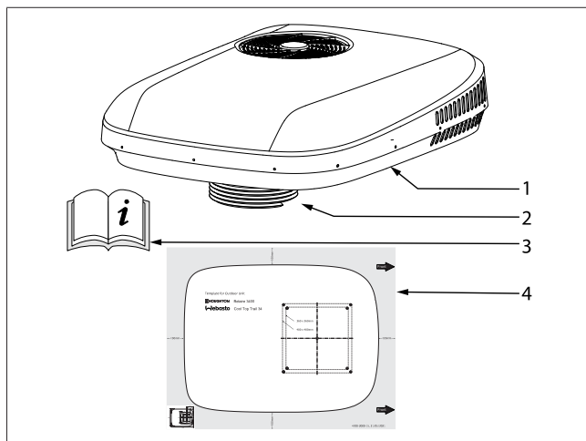
Abb. 1 Außeneinheit
