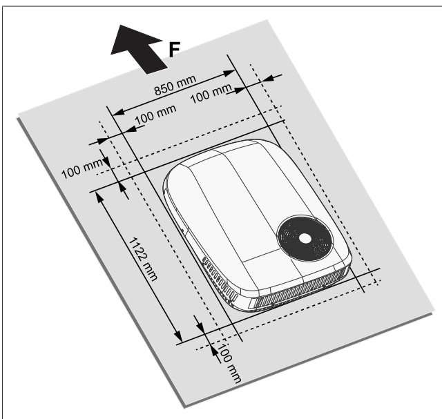
Fig. 5 Sens d'installation de l'unité extérieure
