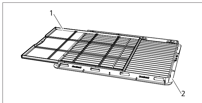
Fig. 56 Filtro dell'aria
