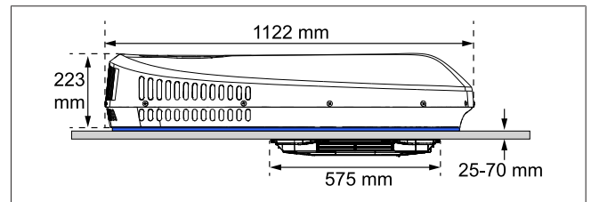
Bild 7 Monteringsmått (vy från sidan)
