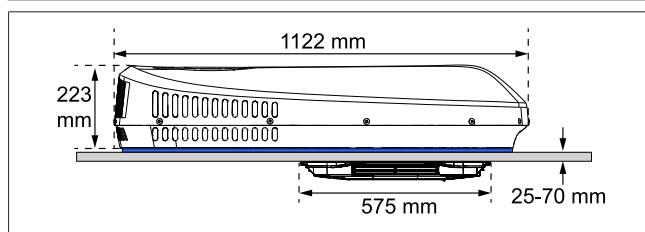
Afb. 7 Montage-afmetingen (zij-aanzicht)
