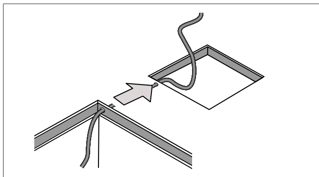
Bild 11 Strömförsörjningskabel
