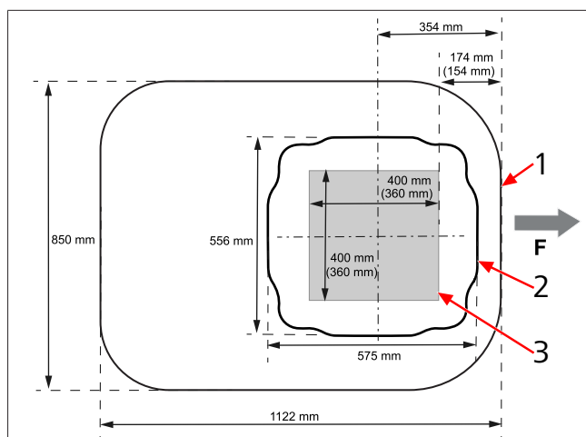
Afb. 6 Montage-afmetingen (boven-/onderaanzicht)
