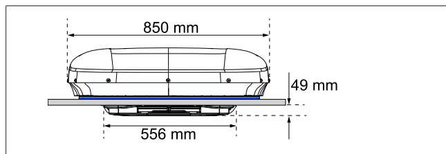
Afb. 8 Montage-afmetingen (vooraanzicht)
