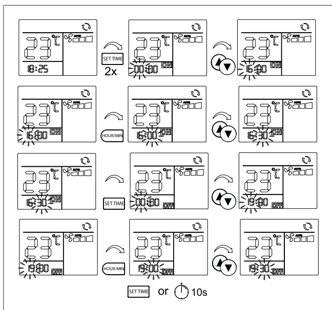
Abb. 45 Timer einstellen
