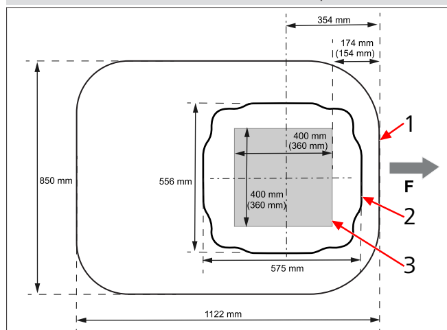
Fig. 6 Mesures pour l'installation (vue du haut/de dessous)
