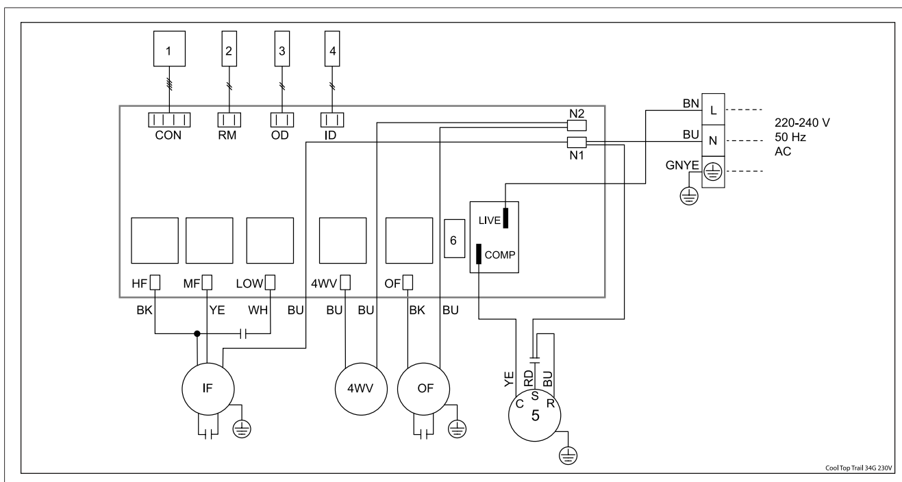
Bild 58 Systemkopplingsschema
