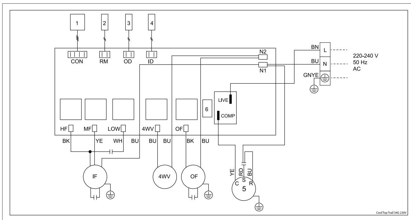
Fig. 58 Esquema eléctrico
