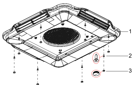
Fig. 30 Fixation du distributeur d'air au plafond
