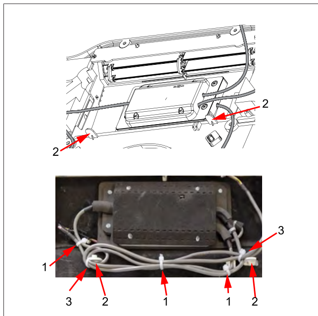
Bild 27 Säkra kablarna
