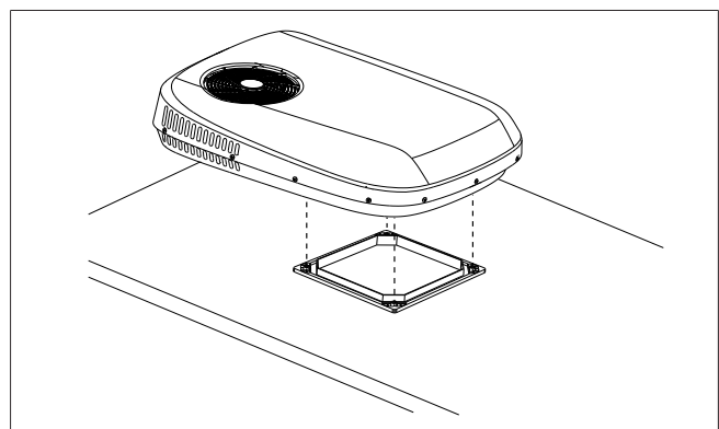
Fig. 18 Posicionamiento de la unidad exterior
