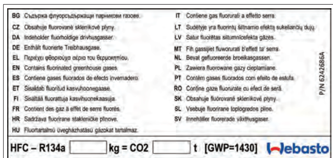
Fig. 17 Autocollant de charge du système en R134a
