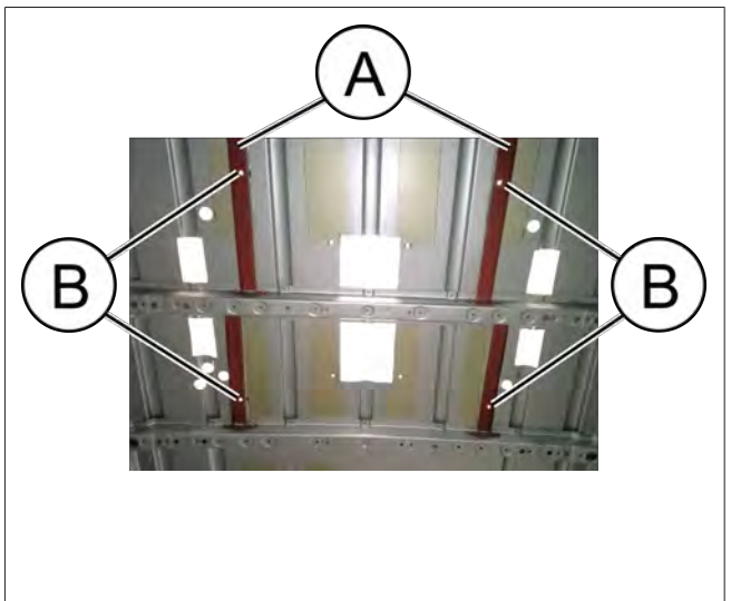
Fig. 5 Cross Beams
