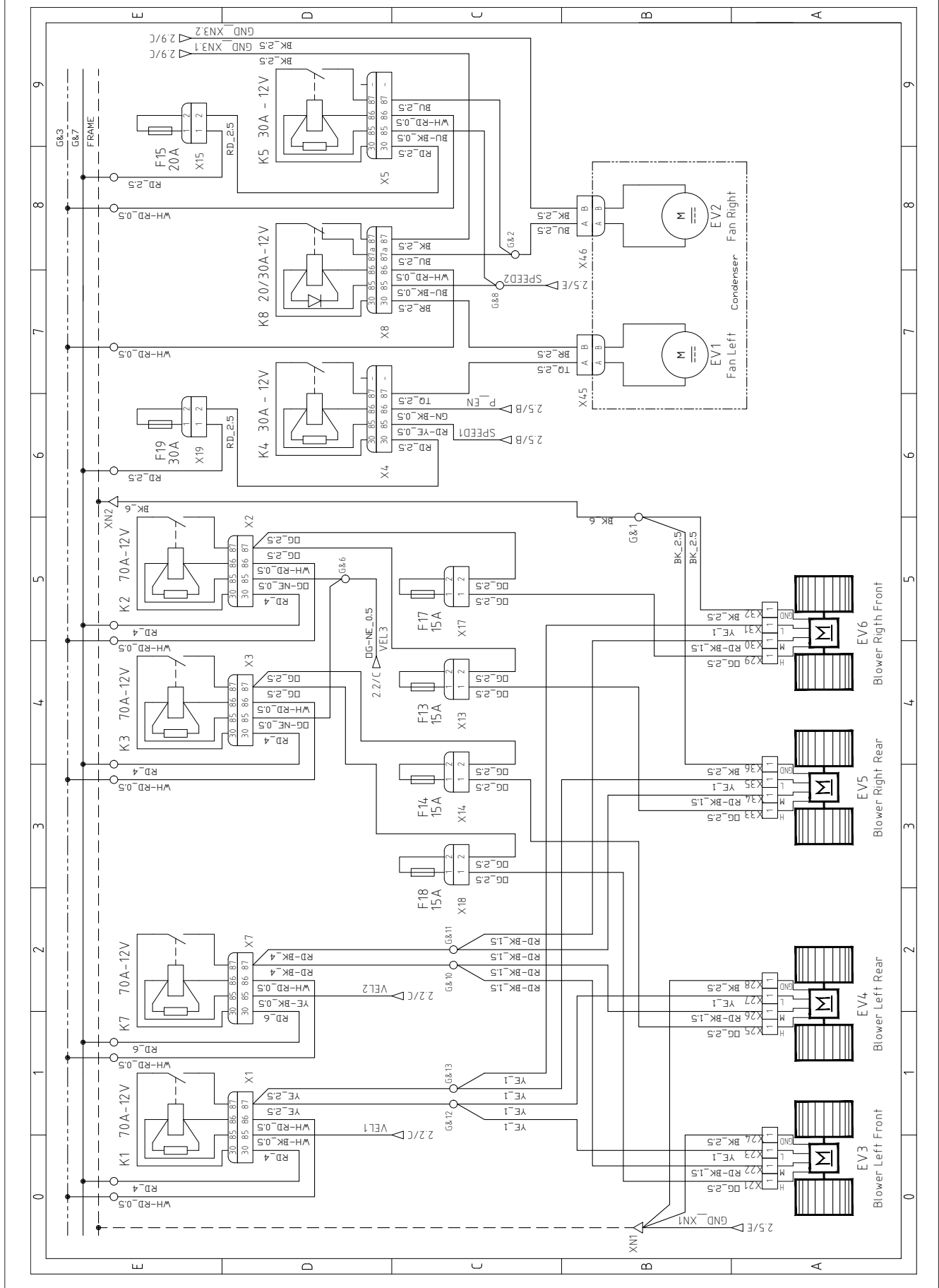
Fig. 24 Circuit électrique
