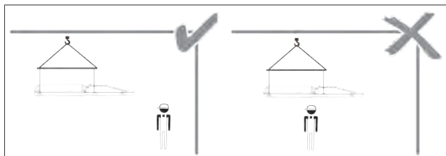
Abb. 2 Es dürfen sich keine Personen unter dem angehobenen Klimaanlage Rahmen aufhalten!
