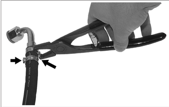
Abb. 22 Schelle festziehen
