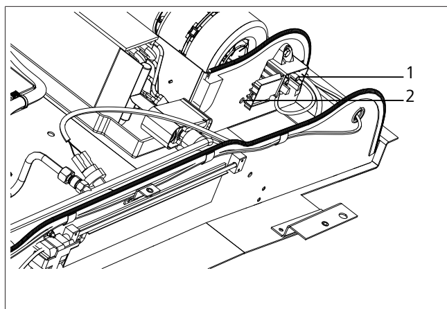
Abb. 13 Stromversorgungskabel
