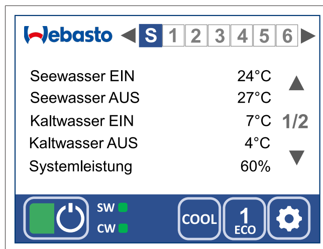
Fig. 3 Affichage système Page 1
